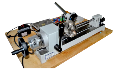
LASER Messvorrichtung für Turbinenschaufeln LASER measuring system for turbine wheels
